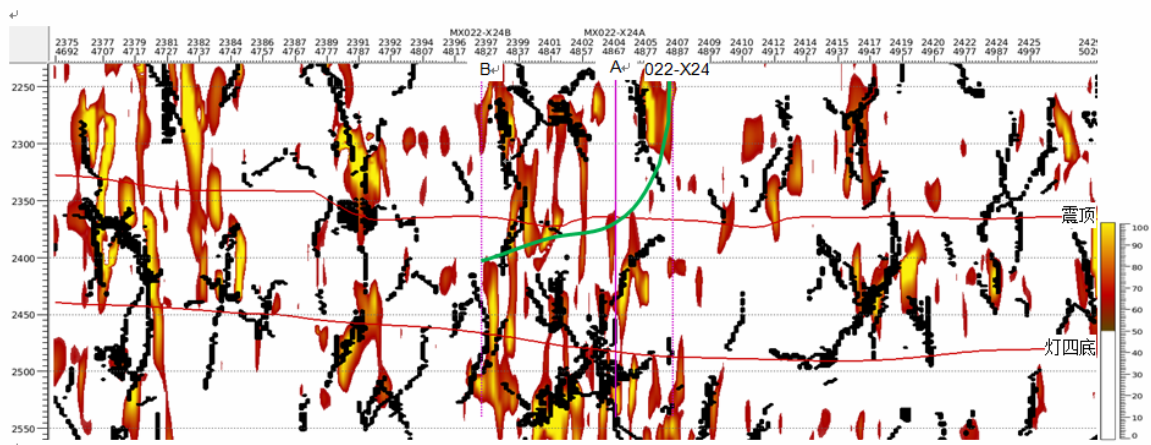
附图6 过磨溪022-X24井轨迹缝洞预测剖面
