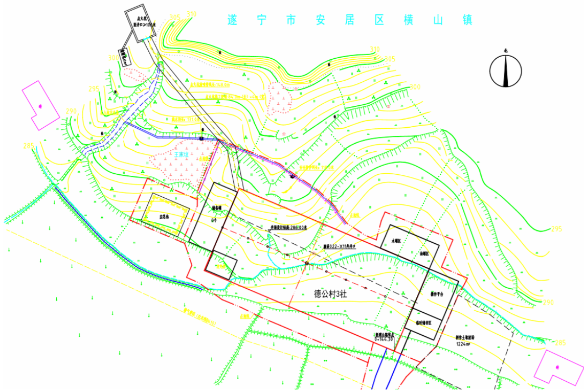
图 3-1 项目平面布局示意图
